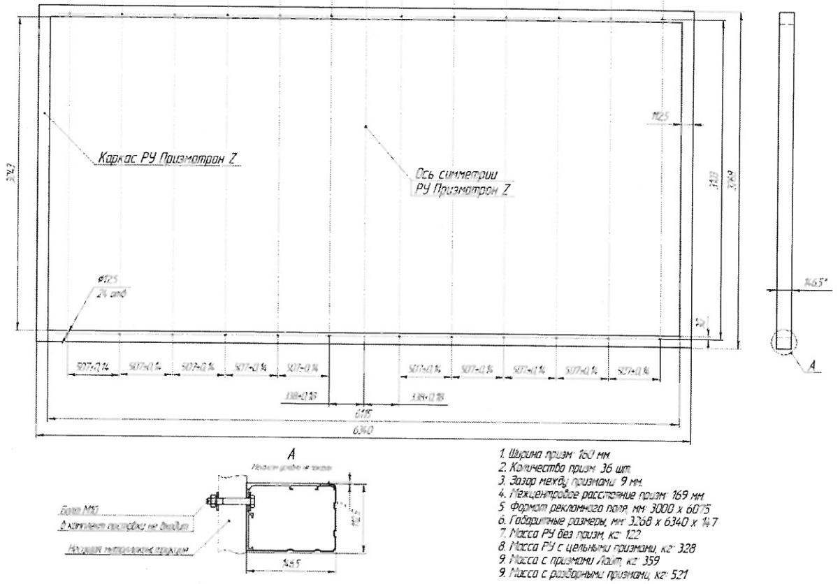
СХЕМА ВЫПОЛНЕНИЯ ПРИСОЕДИНИТЕЛЬНЫХ ОТВЕРСТИЙ В НЕСУЩЕЙ КОНСТРУКЦИИ ДЛЯ РУ ПРИЗМАТРОН Z-3X6X0,16
